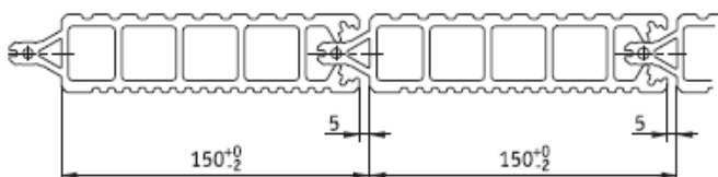
legging med ca. 5 mm fuge = dekning 148 - 150 mm
