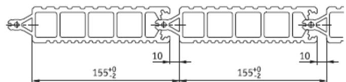
legging med ca. 10 mm fuge = dekning 153 - 155 mm
